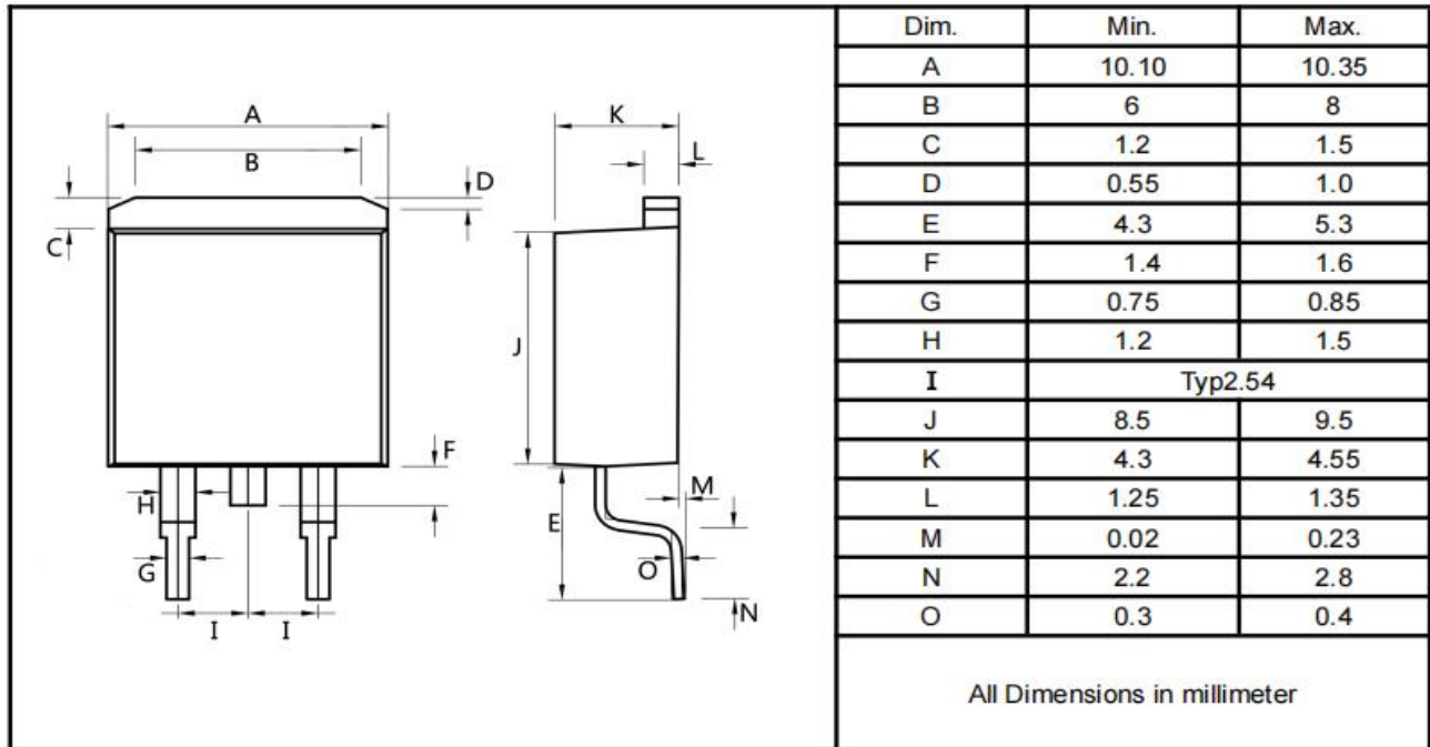
TO-263
